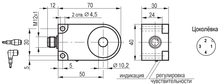
Габаритный чертеж
